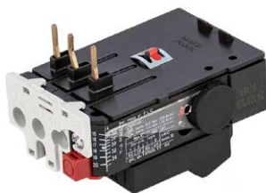
Relé Térmico 24-32 DANFOSS (047H0215)
