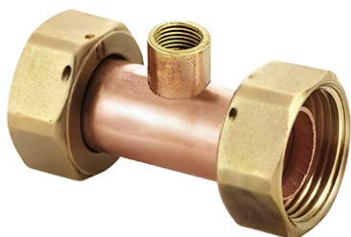
Doble Tuerca De 1 1/2"X2" Con Toma De 1/8"
