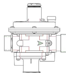
Regulador Fbl04z 130 Con Ps: 90 ÷ 170mbar Montado Para Bg16 Mpa E/S: M 1 1/4" X M 1 1/2"
