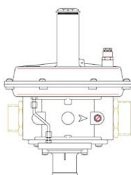
Regulador Rbl06z 160 Con Ps: 150 ÷ 350 Mbar Montado Para Bg25 Mpa E/S: M 1 1/2" X M 2"
