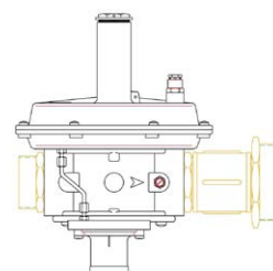
Regulador Rbl07z 130 Con Ps: 32 ÷ 60 Mbar Montado Para Bg65 Mpa E/S: M 2" X M 3"
