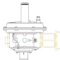
Regulador Rb06z 130 Con Ps: 32 ÷ 60 Mbar Montado Para Bg65 Mpb E/S: M 1 1/4" X M 3"
