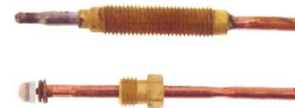
Termopar cabeza roscada M9x1 L=600 mm
