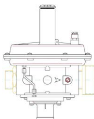
Regulador Rbl06z 130 Con Ps: 32 ÷ 60 Mbar Montado Para Bg40 Mpa E/S: M 1 1/2" X M 2 1/2"
