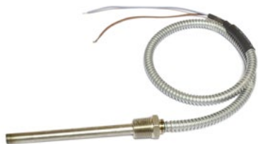
Calefactor De Cartucho Para Compresor Copeland 70w Diam. 10mm Long. 68mm
