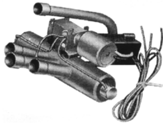
Válvula 4vias inversora modelo SH 20-47 con bobina
