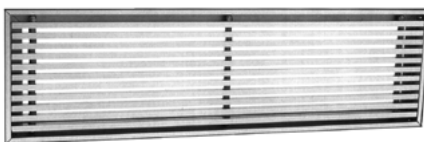
Rejilla lineal de aire con marco 24mm y aletas fijas a 0° MADEL LMT 700x75mm acabado anodizado plata mate
