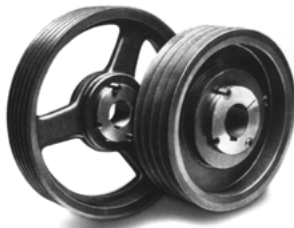
Polea casquillo cónico SPA-A 1 canal Ø315mm
