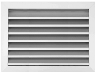
Rejilla retorno de aire aletas fijas 45° MADEL DMT-AR 900x150mm anodizado plata mate
