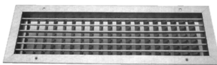
Rejilla impulsión de aire doble deflexión MADEL CMT-AN 350x150mm acabado anodizado plata mate
