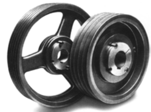
Polea casquillo cónico SPB-B 1 canal Ø200mm
