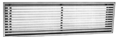
Rejilla lineal de aire con marco 24mm y aletas fijas a 0° MADEL LMT 200x100mm acabado anodizado plata mate
