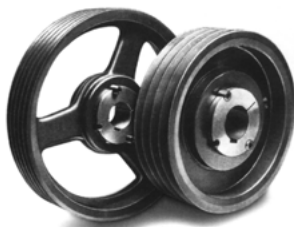
Polea casquillo cónico SPB-B 2 canales Ø160mm
