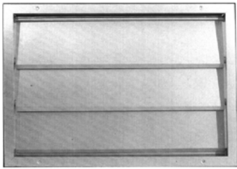
Compuerta de sobrepresión MADEL SMG 800x600mm montaje en conducto de chapa
