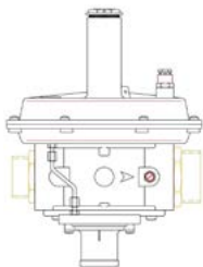
Regulador Rbl06z 160 Con Ps: 150 ÷ 350 Mbar Montado Para Bg25 Mpa E/S: M 1 1/2" X M 2"
