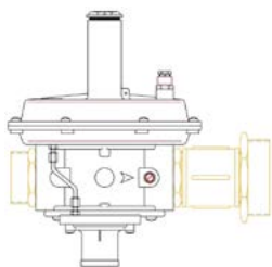
Regulador Rb107z 150 Con Ps: 85 ÷ 180 Mbar Montado Para Bg65 Mpa E/S: M 2" X M 3"
