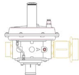
Regulador Rbl07z 130 Con Ps: 32 ÷ 60 Mbar Montado Para Bg65 Mpa E/S: M 2" X M 3"
