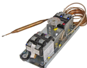
Termostato 4 etapas A36
