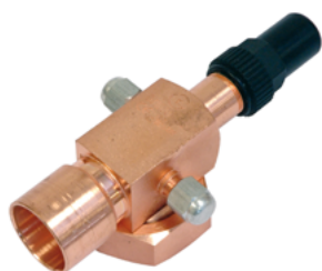
Valvula De Servicio Rotalock Entrada 1-3/4" Roscar, Salida 2-1/8" Soldar(Recomendable Uso De Hf07020 Masilla Protectora)
