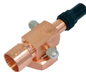
Valvula De Servicio Rotalock Entrada 1-3/4" Roscar, Salida 1-5/8" Soldar(Recomendable Uso De Hf07020 Masilla Protectora)
