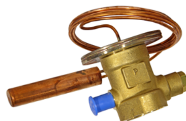
Elemento termostático ALCO XB1019MW55-1B con capilar de 1,5m
