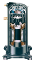
Compresor Scroll Zp-61-Kce R-410a 420v Iii/50 Soldar
