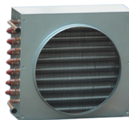
Condensador HISPANIA de aire forzado sin ventilador HCA-114 11x4 tubos
