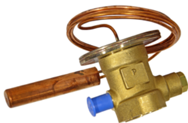
Elemento termostático ALCO XC726HW35-2B con capilar de 3m
