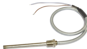
Calefactor De Cartucho Para Compresor Copeland 70w Diam. 10mm Long. 112mm
