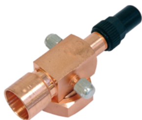
Valvula De Servicio Rotalock Entrada 1" Roscar, Salida 5/8" Soldar(Recomendable Uso De Hf07020 Masilla Protectora)
