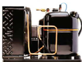
Unidad Condensadora L'Unité Hermetique Caj2446z R404a (220v-60hz) (V120.13/T60)
