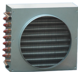
Condensador HISPANIA de aire forzado sin ventilador HCA-84 8x4 tubos
