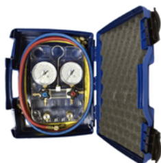
Kit de carga con analizador WIGAM K-SPY2PFA4-5-GYSS60-LV PARA R22, R134a, R404A y R407C
