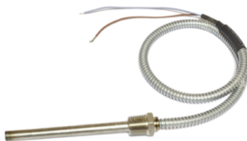
Calefactor De Cartucho Para Compresor Copeland 70w Diam. 10mm Long. 68mm
