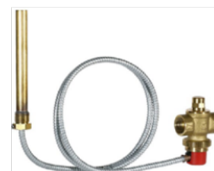
Valvula de seguridad termica HONEYWELL TS-131 Rosca 3/4" hembra, capilar 1300mm, abre y descarga el agua a 95°C
