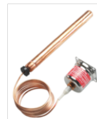
Carga univ. sensor d. 18x210mm + 25 + 65 capilar 2m 003N0078
