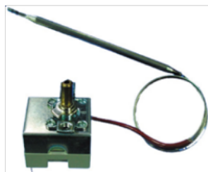
Termostato bulbo y capilar CAMPINI TY95 Escala 0a 40°C ,capilar 1 metro , contacto conmutado
