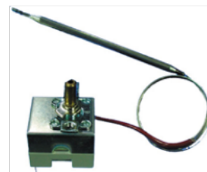
Termostato con bulbo y capilar CAMPINI TY95 bulbo y capilar Escala -35/+ 35,Capilar 1,5 mts.Bulbo diam 6 x88mm cobre
