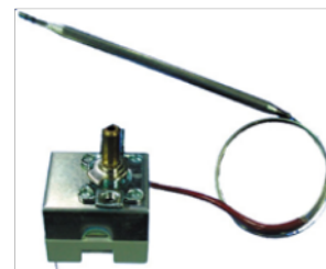
Termostato bulbo y capilar CAMPINI TY95 Escala 0/+ 120°C .Capilar 1 metro . Bulbo diam 6 x88mm cobre
