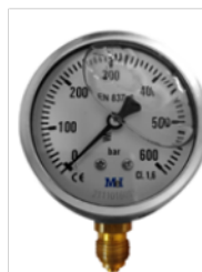
Manómetro glicerina MEI Ø63mm vertical 1/4" 0 a 600bar
