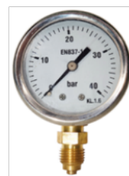
Manómetro con glicerina diámetro 50 mm vertical rosca 1/4" 0-40 bar
