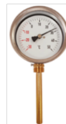
Termómetro bimetalico diámetro 80 mm vertical longitud 100 mm con vaina rosca 1/2" -30 a +50 °C.
