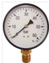
Manómetro diam. 100 mm. VERTICAL rosca 1/2" 0-60 bar
