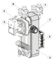
Intercambiador de placas SONNENKRAFT FWSS S2
