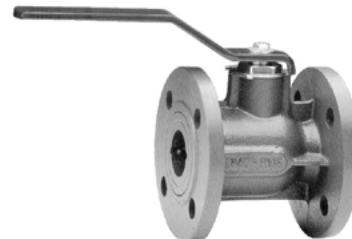
Válvula de bola, cuerpo de hierro, bola de latón, PN16, con bridas DN-40
