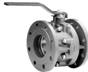
Válvula de bola, cuerpo de hierro, bola de latón, PN16 , con bridas DN-150
