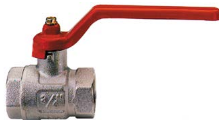
Válvula de bola de latón hembra-hembra, rosca 1/4"
