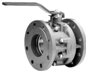
Válvula de bola, cuerpo de hierro, bola de latón, PN16 , con bridas DN-100
